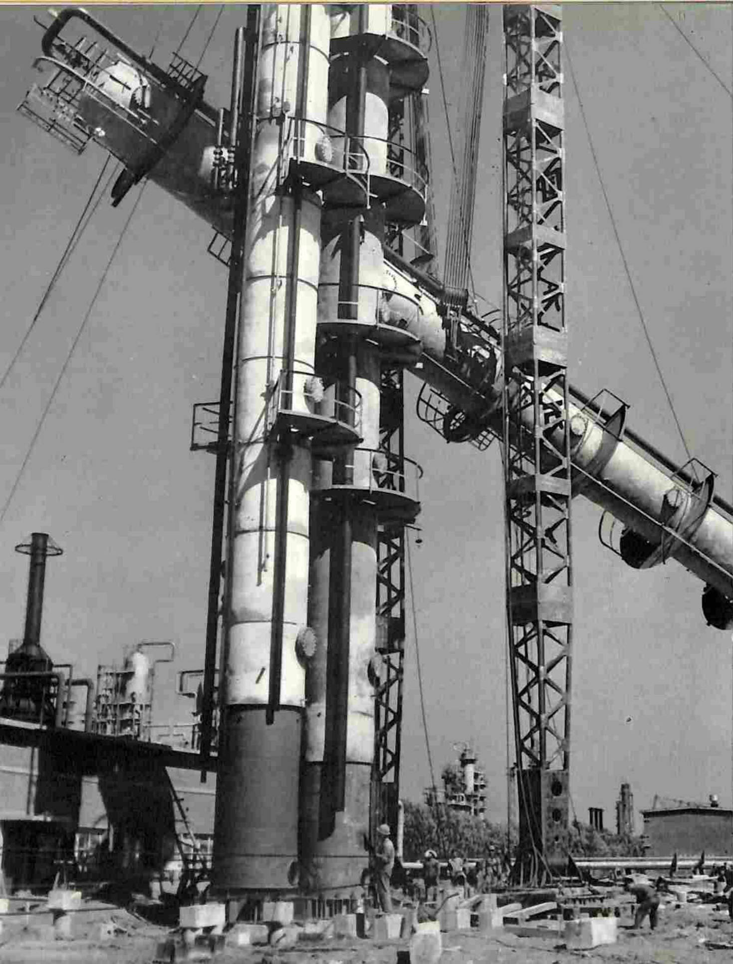
炼塔吊装
