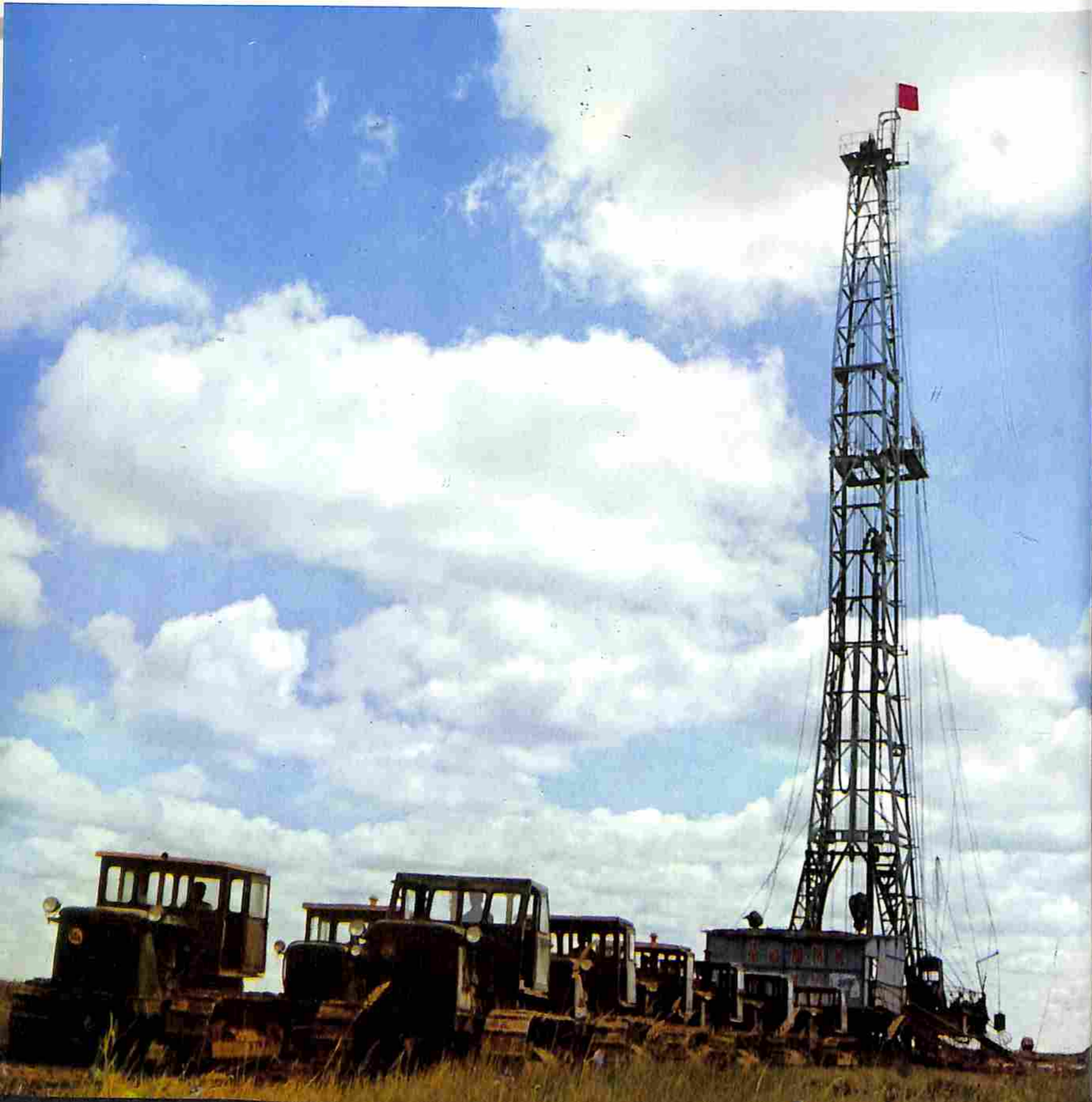
钻机整体搬家
