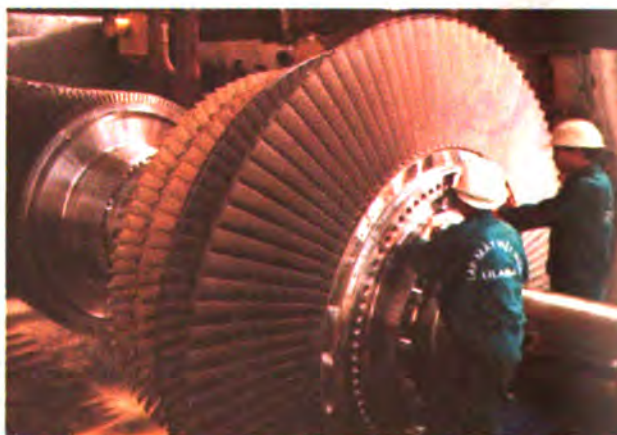
Lắp Tuabin hơi - Nhà máy Nhiệt điện Phú Mỹ
