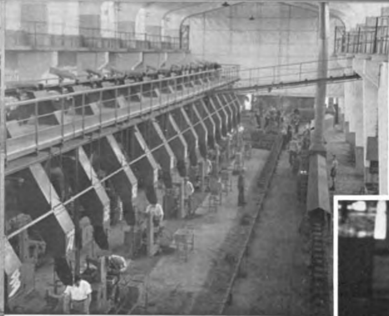
上海机械制造工业能自制各种大型机械和精密复杂的仪器。左图是中国纺织机器厂的自动化皮带送砂机。
